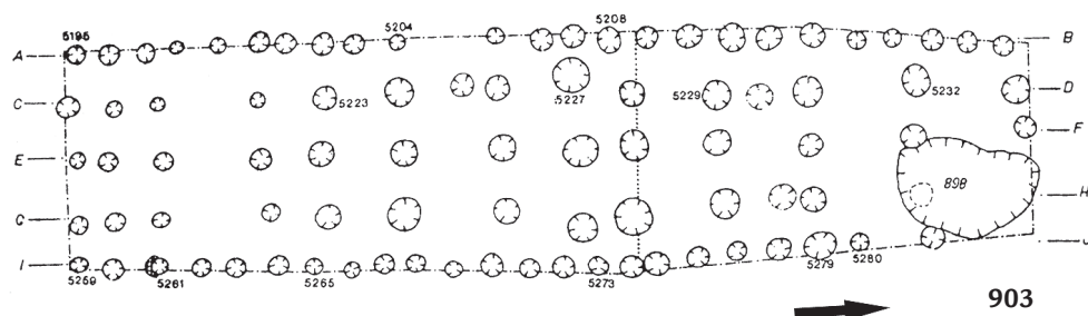
■ Obr. 3 Půdorys domu 903 mladšího stupně LnK na sídlišti v Bylanech u Kutné Hory. Podle Pavlů et al. 1985, 16.
